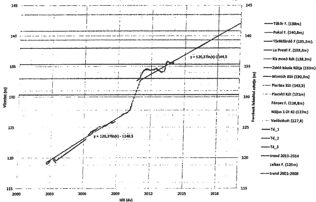
3. ábra: A tatabányai karsztvíz megfigyelő kutak vízszintjének változása és a vízszint alakulásának előrejelzése (a vízszintes vonalak a források fakadási szintjeit jelzik; a szaggatott vonal adathiányt jelöl)
